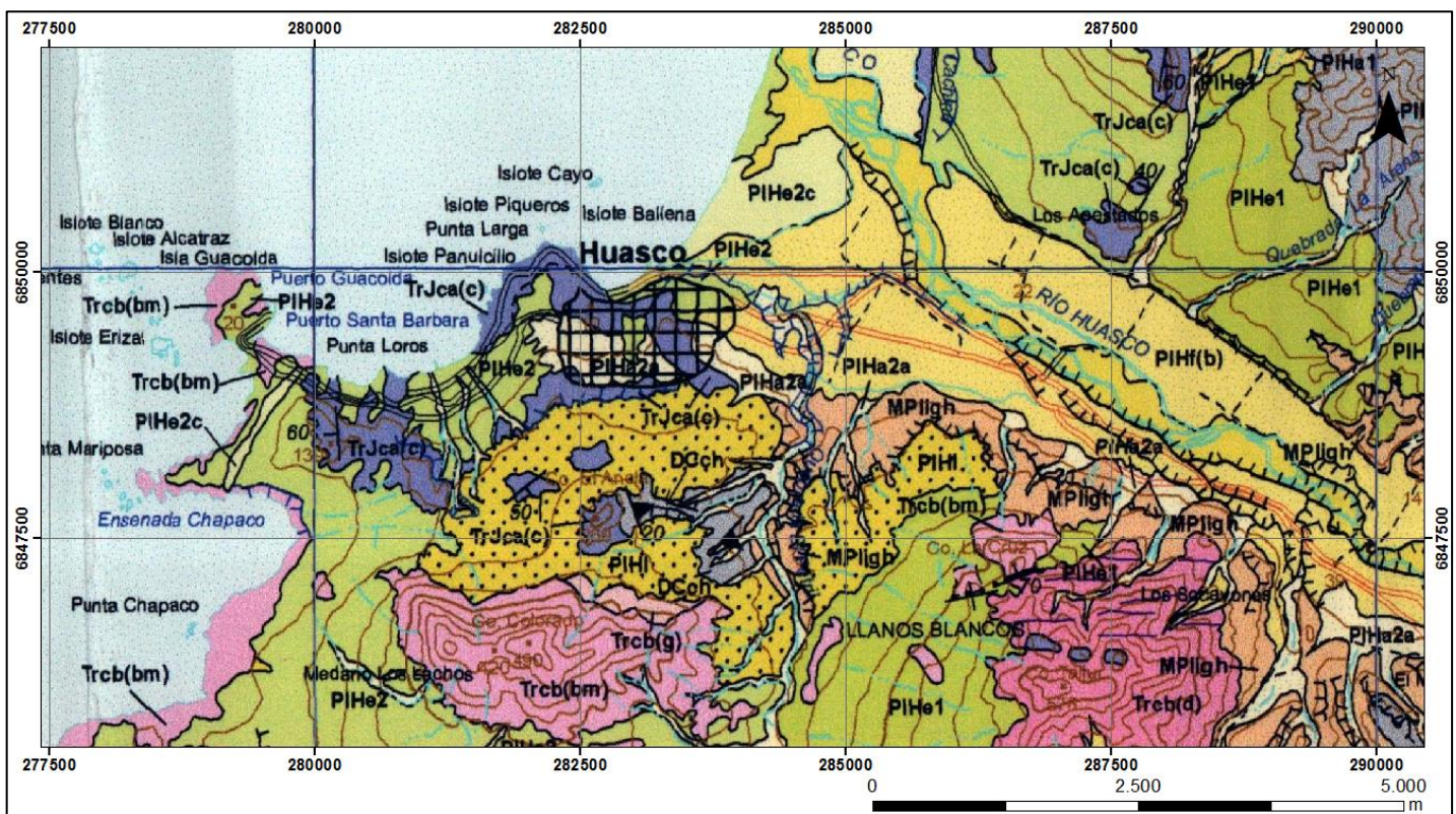
Figura 3. Mapa Geológico del área de estudio (Cuadro Rojo). DCch: metaarenitas cuarcíferas y esquistos cuarzo-micáceos del Complejo Epimetamórfico Chañaral, de edad Devónico - Carbonífero inferior. Trcb: granitos del Complejo Intrusivo Carrizal Bajo del Triásico. TrJca: secuencia marina clástica y volcánica de la Formación Canto del Agua de edad Anisico - Sinemuriano. MPLigh: gravas con fragmentos redondeados correspondientes a las Gravas del río Huasco. PIHa2a: depósitos aluviales, PIHe2: depósitos eólicos. PIHf: Depósitos fluviales.
