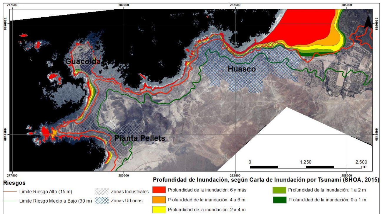
Figura 7. Mapa de Riesgo de Tsunami en el área de Huasco. Se destaca el mapa de inundación por tsunami del SHOA (2015), pero se consideraron escenarios extremos con zonas con cotas entre 15 y 30 m.s.n.m. Mapa de elaboración propia.
