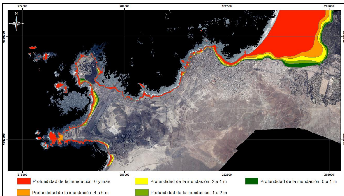
Figura 6. Mapa de Inundación por Tsunami, versión 2015, elaborado por el Servicio Oceanográfico de la Armada de Chile (SHOA).
