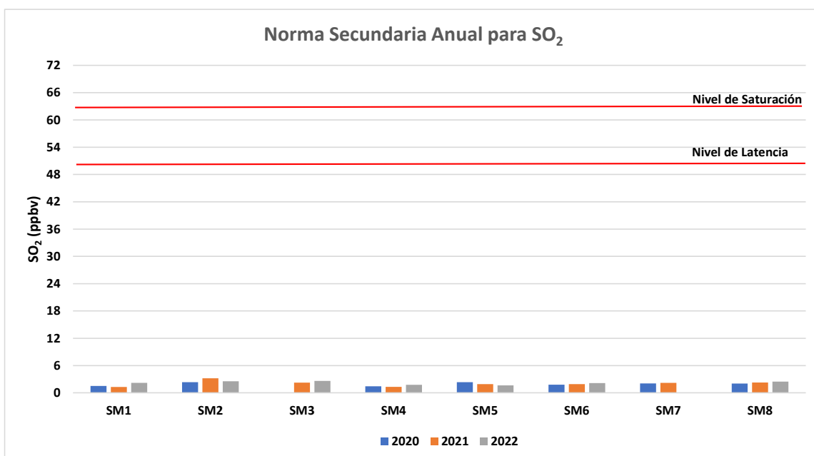
Gráfico 11 Norma secundaria anual para SO 2 , período 2020 al 2022
