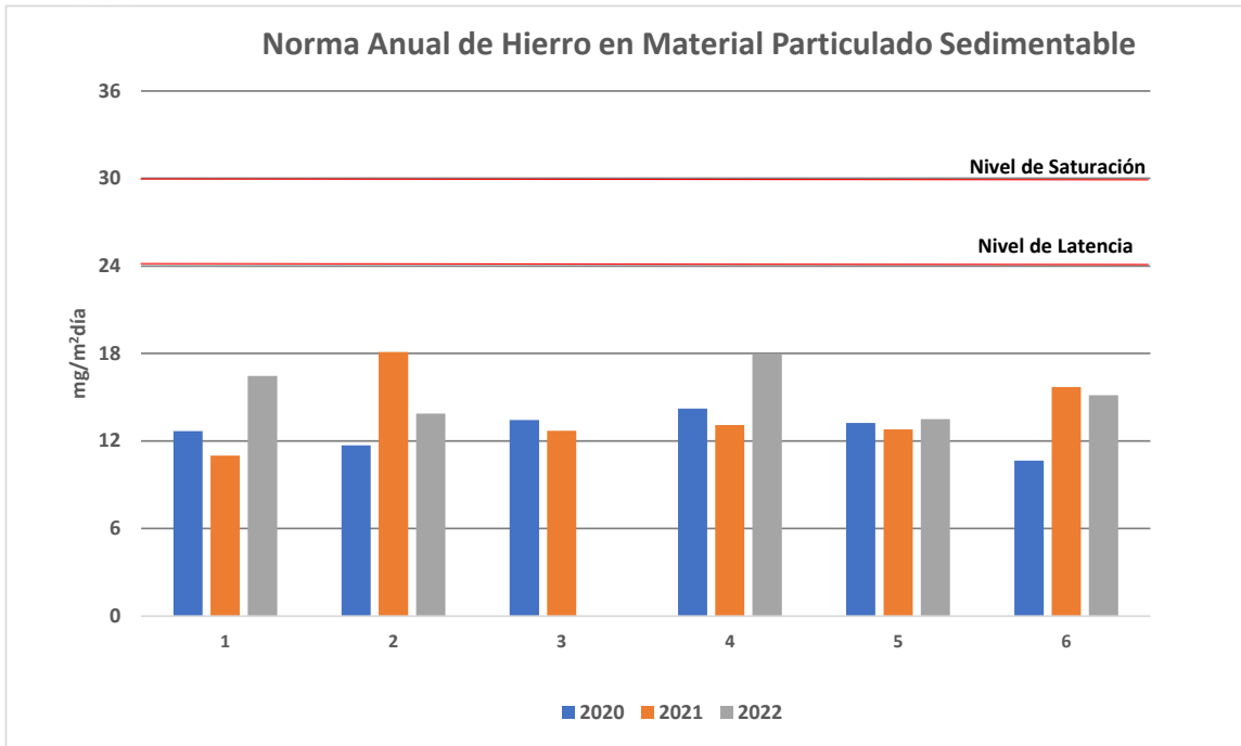
Gráfico 16 Concentración anual de MPS para los años 2020, 2021 y 2022
