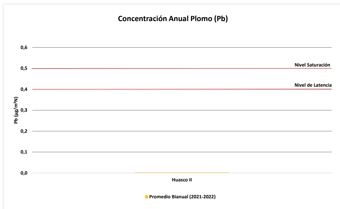
Gráfico 5 Norma anual para Pb, promedio bianual período 2021 al 2022
