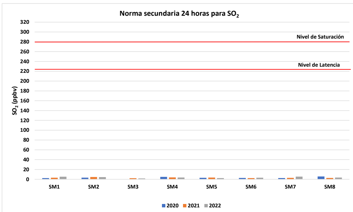
Gráfico 9 Norma secundaria 24 horas para SO 2 , período 2020 al 2022
