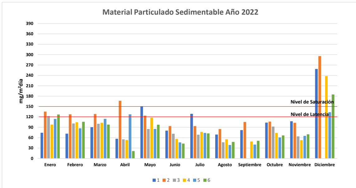
Gráfico 14 Concentración mensual de MPS para el año 2022
