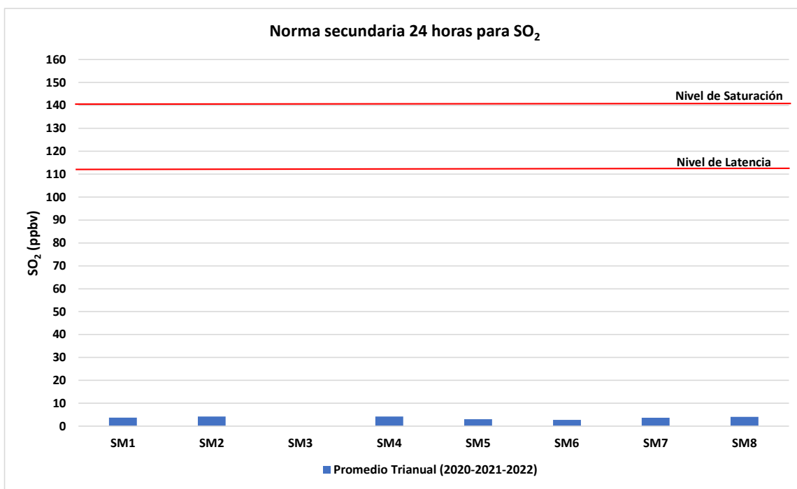
Gráfico 8 Norma secundaria 24 horas para SO 2 , promedio trianual período 2020 al 2022
