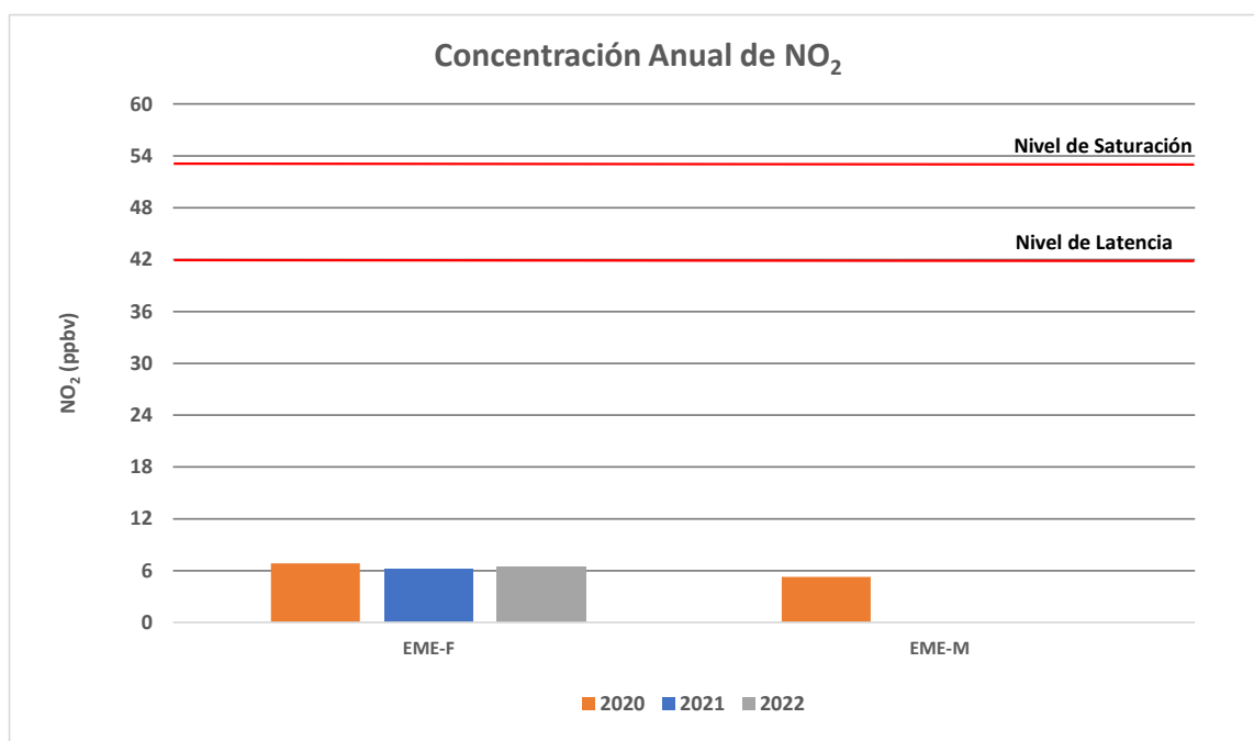
Gráfico 4 Concentración anual para NO 2 , periodo 2020 al 2022
