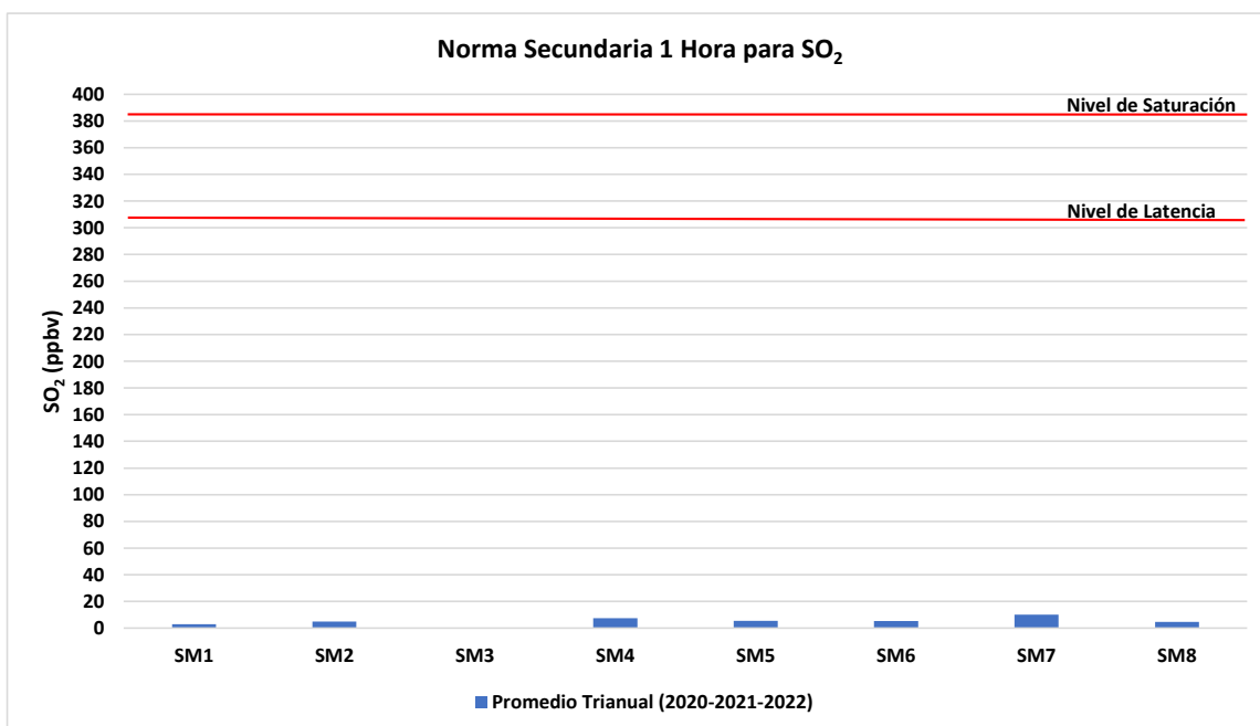
Gráfico 6 Norma secundaria 1 hora para SO 2 , promedio trianual durante el período 2020 al 2022
