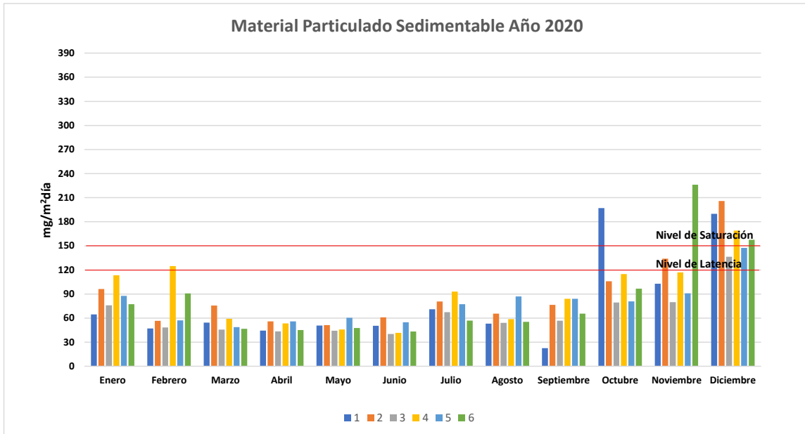
Gráfico 12 Concentración mensual de MPS para el año 2020
