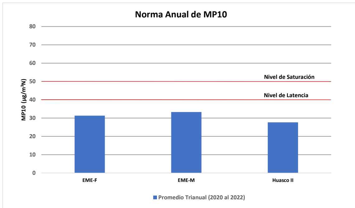
Gráfico 2. Norma anual para MP10, promedio trianual periodo 2020 al 2022
