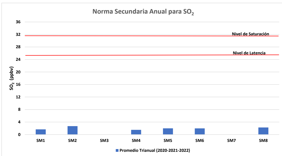
Gráfico 10 Norma secundaria anual para SO 2 , promedio trianual período 2020 al 2022
