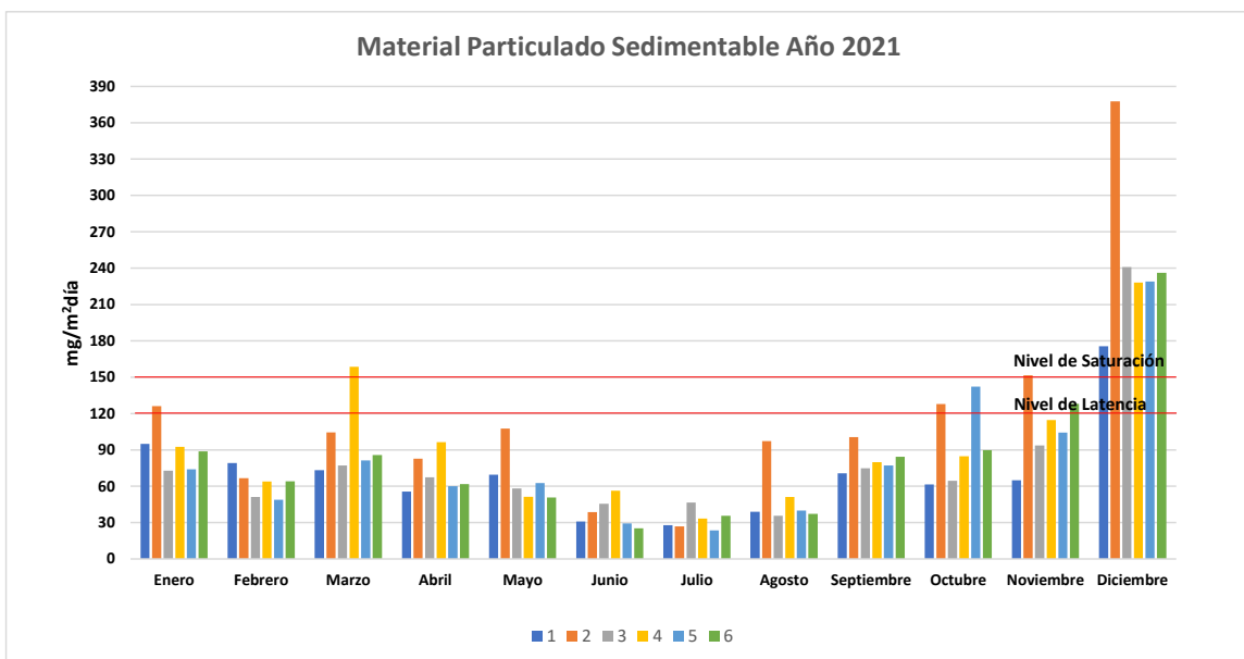
Gráfico 13 Concentración mensual de MPS para el año 2021
