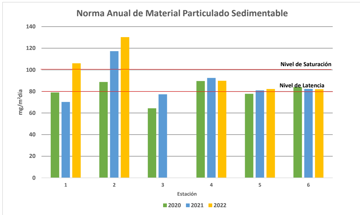
Gráfico 15 Concentración anual de MPS para los años 2020, 2021 y 2022
