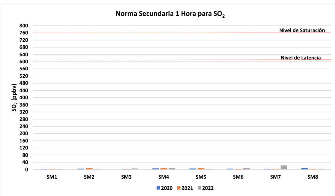
Gráfico 7 Norma secundaria 1 hora para SO 2 , período 2020 al 2022
