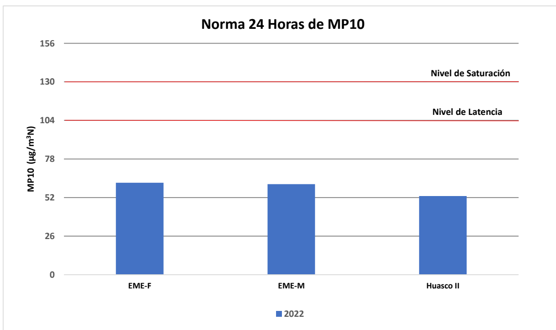
Gráfico 1 Norma 24 horas para MP10 para el año 2022
