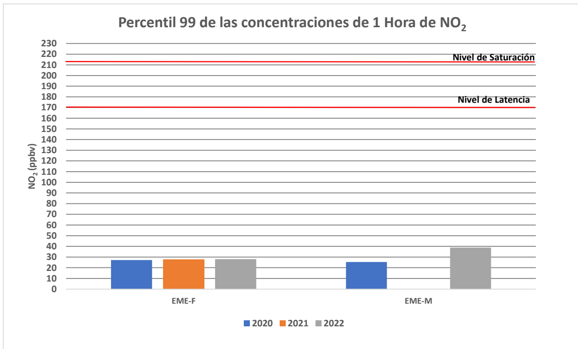
Gráfico 3 Percentil 99 de las concentraciones de 1 hora para NO 2 , período 2020 al 2022
